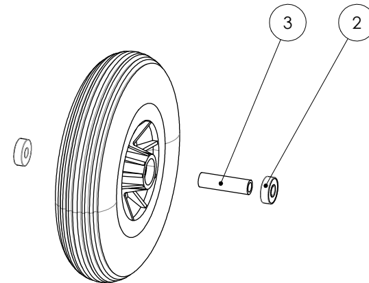
Länkhjul 8" solid svart - 7350006080272
